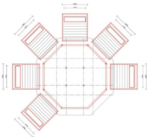
Plattegrond met zij-schutpanelen
