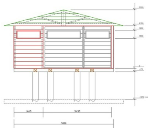
Vooraanzicht (vanaf dijk)
